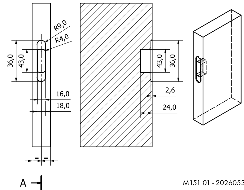
frézování zárubně
